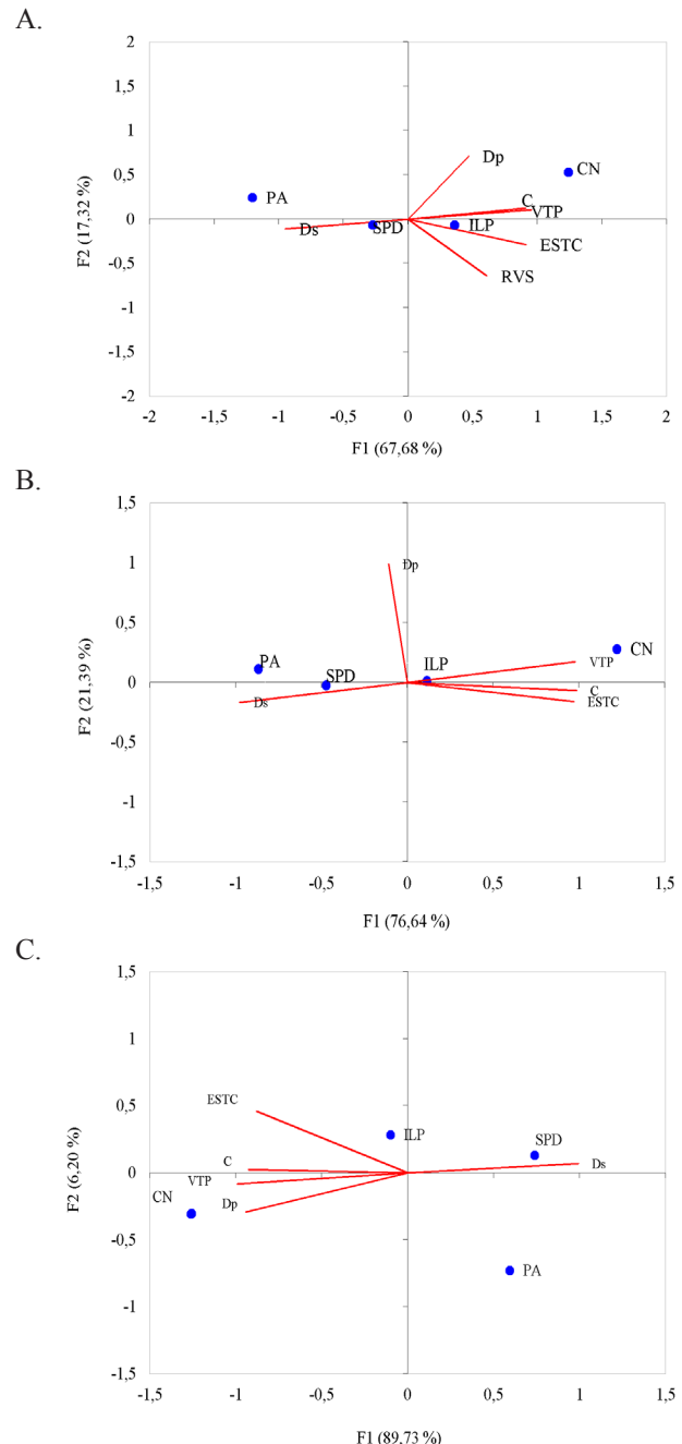
Figura 2. Diagramas de ordenação produzidos por análise de componentes principais, das características avaliadas em amostras de solo coletadas na camada de 0-5 cm (A), 5-10 cm (B) e 10-20 cm (C)
