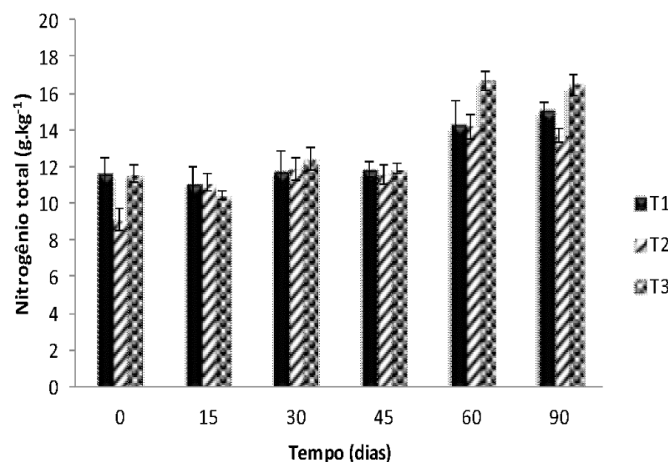
Figura 4. Evolução dos teores de N-total ao longo do processo de compostagem de resíduos de poda de mangueira, jurema-preta ou algarobeira, misturados com esterco bovino e MB-4, na região semiárida do NE do Brasil. T 1 : poda de mangueira, esterco bovino e MB-4; T 2 : poda de jurema-preta, esterco bovino e MB-4 e T 3 : poda de algaroba, esterco bovino e MB-4
