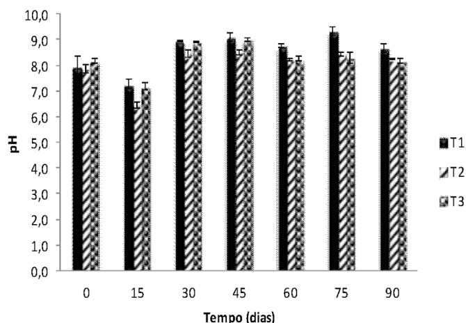
Figura 2. Evolução do pH ao longo do processo de compostagem de resíduos de podas de mangueira, jurema-preta ou algarobeira, misturados com esterco bovino e MB-4, na região semiárida do NE do Brasil. T 1 : poda de mangueira, esterco bovino e MB-4; T 2 : poda de jurema-preta, esterco bovino e MB-4 e T 3 : poda de algaroba, esterco bovino e MB-4
