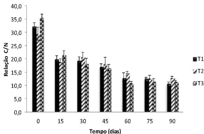
Figura 5. Dinâmica da relação C/N na compostagem de resíduos de poda de mangueiras, jurema-preta, algarobeira, esterco bovino e MB-4 no semiárido NE Brasil. T_1 : poda de mangueira, esterco bovino e MB-4; T_2 : poda de jurema-preta, esterco bovino e MB-4 e T_3 : poda de algaroba, esterco bovino e MB-4
