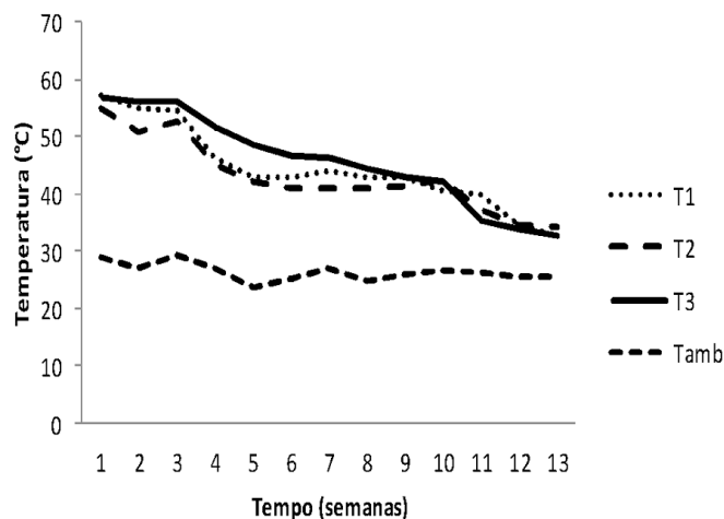
Figura 1. Dinâmica da temperatura ao longo do processo de compostagem de resíduos de podas de mangueira, jurema-preta ou algarobeira, misturados com esterco bovino e MB-4, na região semiárida do NE do Brasil. T 1 : poda de mangueira, esterco bovino e MB-4; T 2 : poda de jurema-preta, esterco bovino e MB-4 e T 3 : poda de algarobeira, esterco bovino e MB-4
